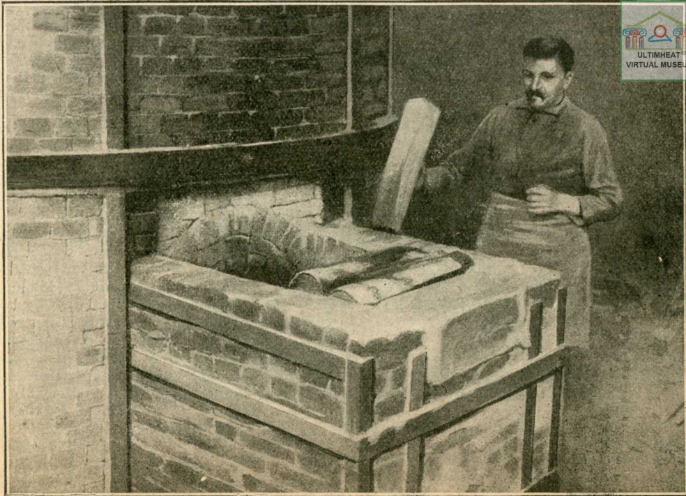
FOYER A COMBUSTION RENVERSEE (ALANDIER) D'UN FOUR A CUIRE LA PORCELAINE
